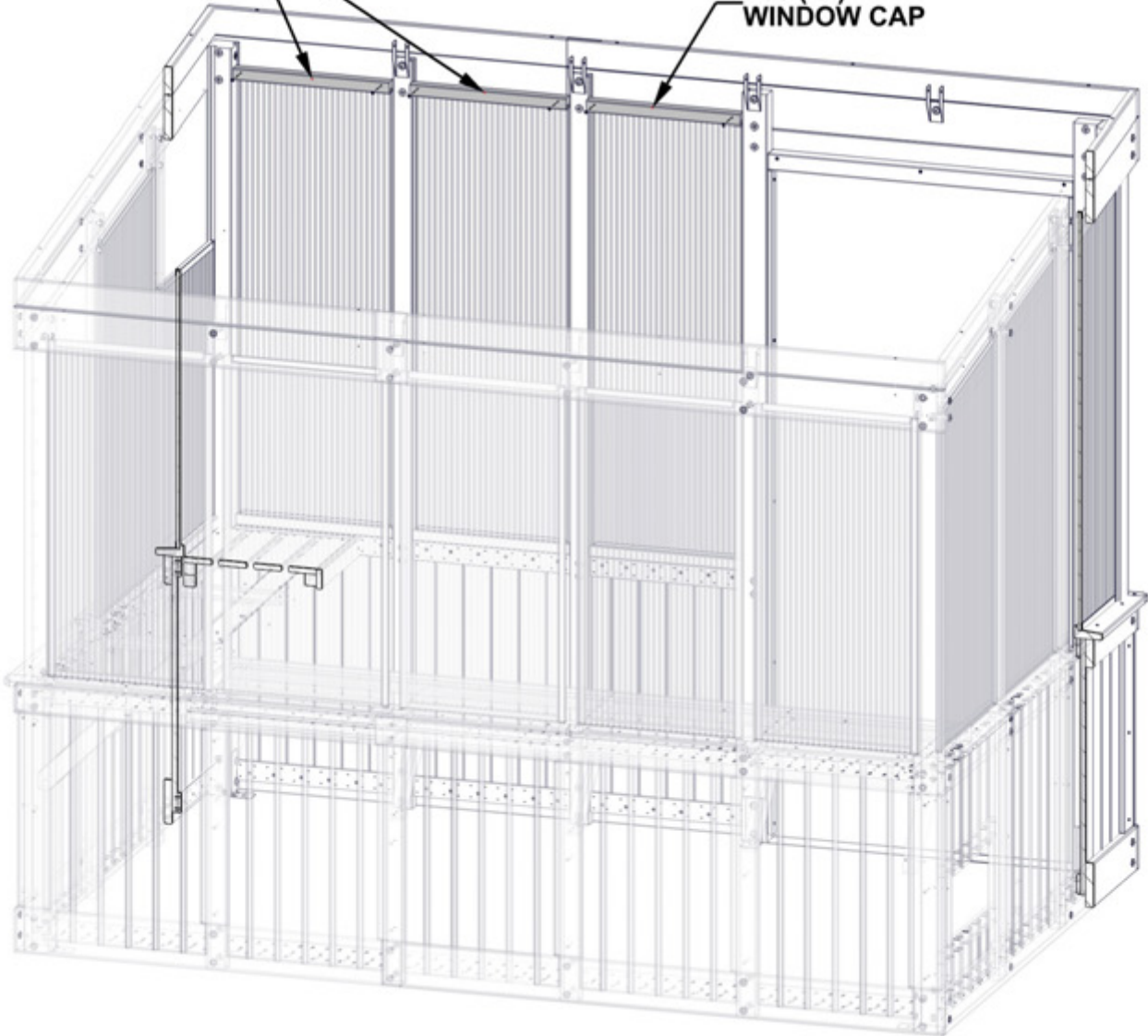
P02 (x2) WINDOW CAP
