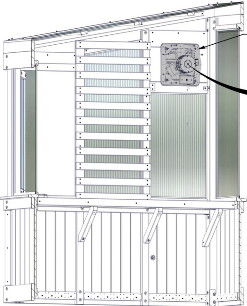
3475 (x1) EXHAUST FAN
