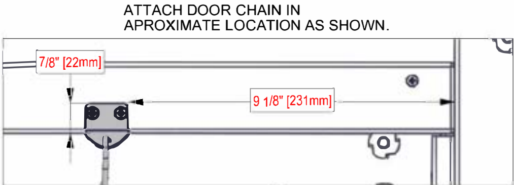
2411 (x1) DOOR PROTECTOR CHAIN
