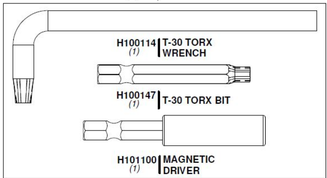
9220119 | TOOL KIT (1)
